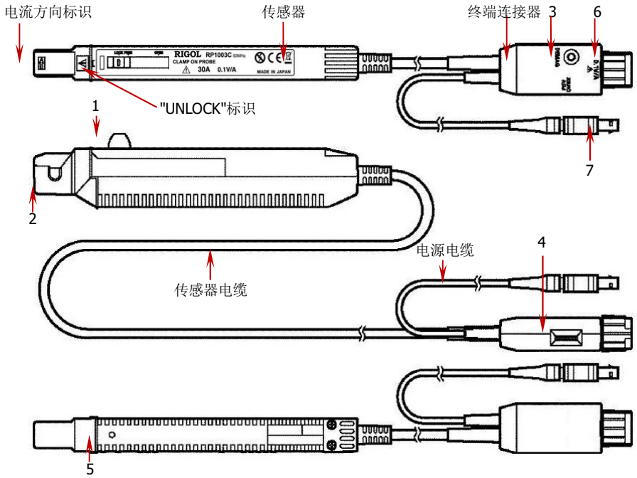
图 1 RP1003C/RP1004C 部件示意图
